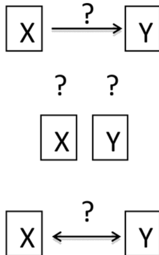
Figura 1 . Representación del método correlacional. Se representa mediante las variables una relación entre dos variables
