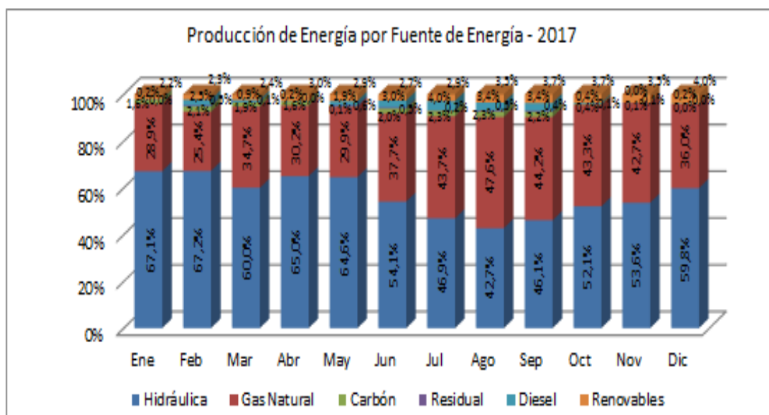
Gráfico N° 02: Producción por fuente de energía
