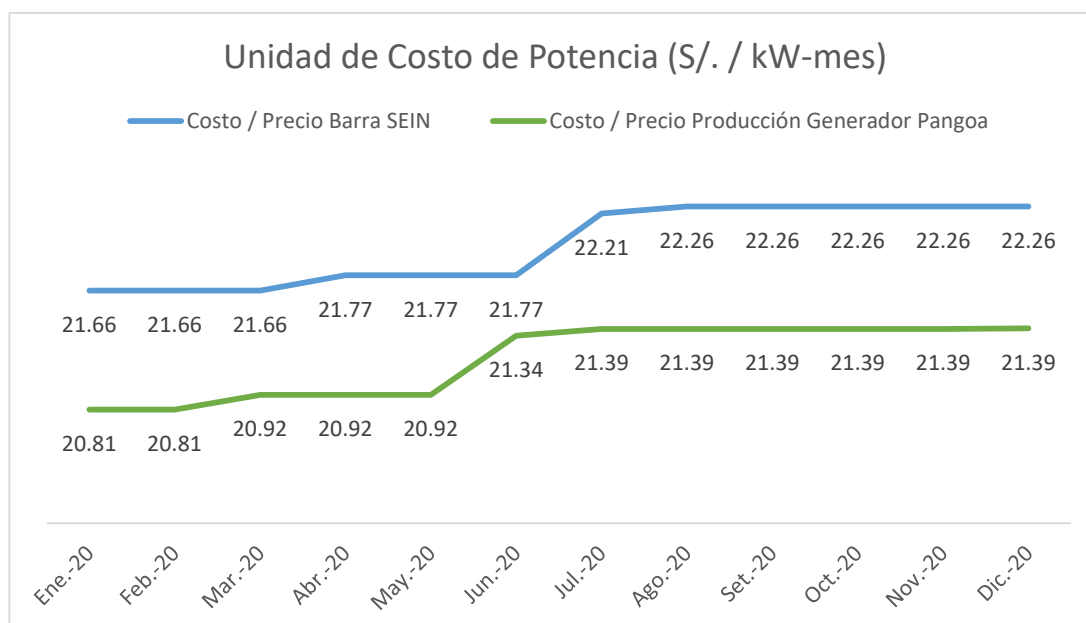
Gráfico N° 11: Indicador comparación del costo fijo de producción de la hidroeléctrica Pangoa y su relación con el precio de potencia en barra del SEIN en la empresa EGEPISA, 2020
