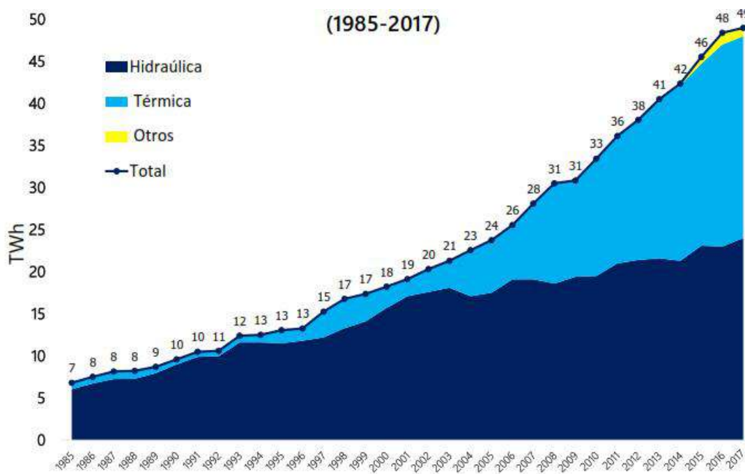
Gráfico N° 01: Producción de la energía eléctrica
