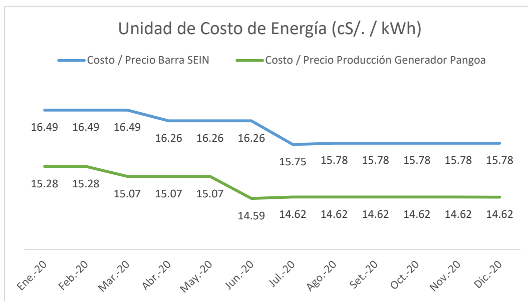
Gráfico N° 12: Indicador comparación del costo variable de producción de la hidroeléctrica Pangoa y su relación con el precio de energía en barra del SEIN en la empresa EGEPSA, 2020
