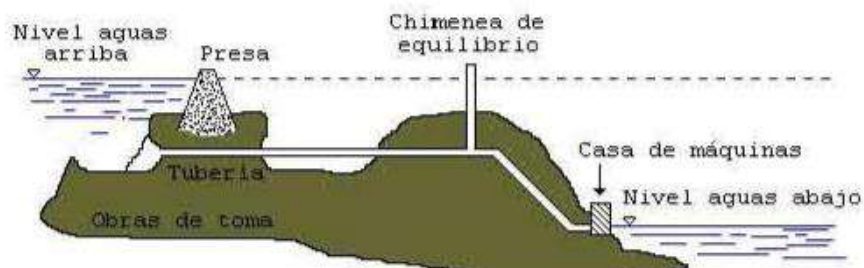
Gráfico N° 03: Esquema típico de hidroeléctrica con presa.
