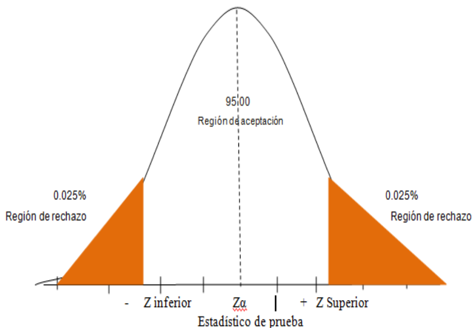
Figura 1. Campana de Gauss de la Hipótesis General
