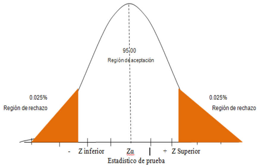
Figura 16. Campana de Gauss de la Hipótesis Específica 2
