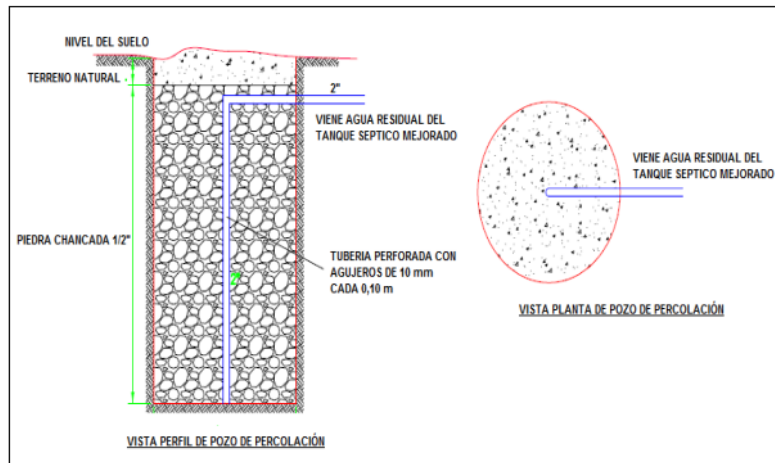
Figura N°05. Vista en planta y corte del pozo del pozo de percolación con relleno de grava de 1/2". Fuente: Norma técnica de diseño: Guía de opciones tecnológicas para sistemas de abastecimiento de agua para consumo humano y saneamiento en el ámbito rural (2018).
