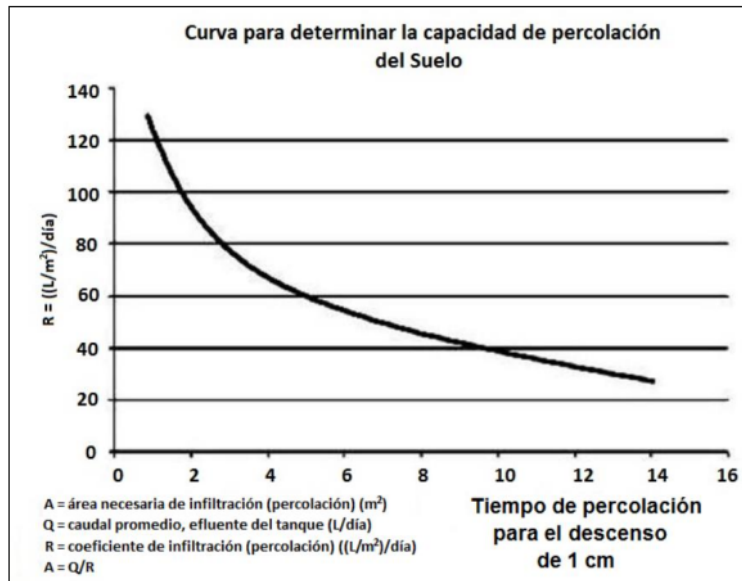
Figura N° 06: Grafico para la determinación de la capacidad de percolación del suelo.
