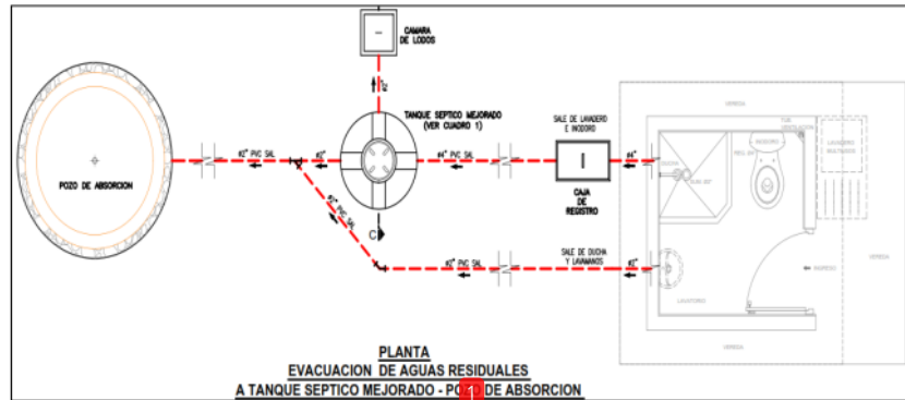
Figura N°07. Vista en planta de los componentes de la UBS con arrastre hidráulico.
