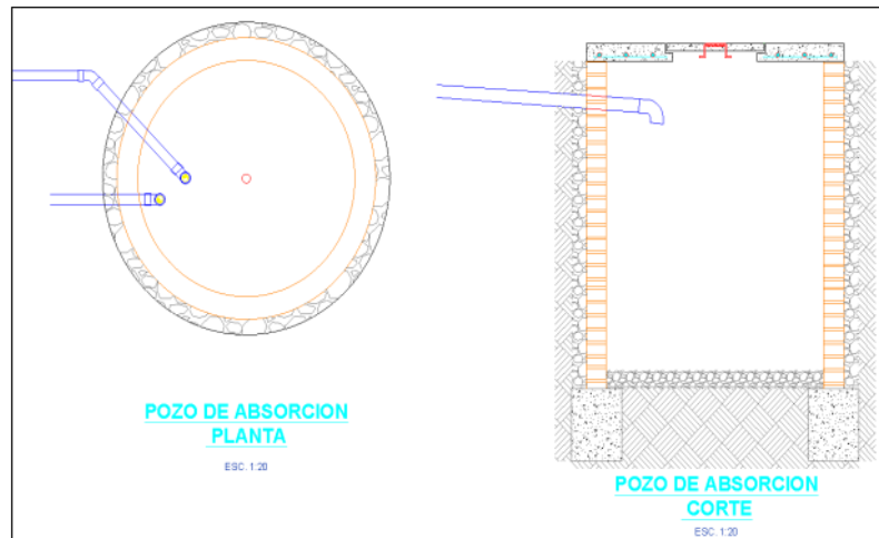
Figura N°02. Vista en planta y corte de pozo de absorción con paredes de mampostería. Fuente: Norma técnica de diseño: Guía de opciones tecnológicas para sistemas de abastecimiento de agua para consumo humano y saneamiento en el ámbito rural (2018).
