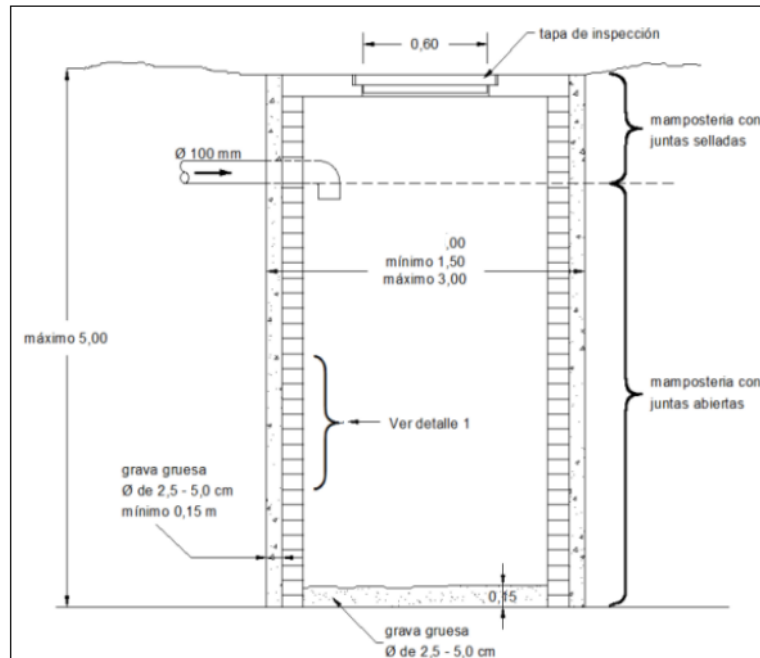
Figura N°04: Componentes del pozo de percolación. Fuente : Reglamento nacional de edificaciones, Norma IS 020.
