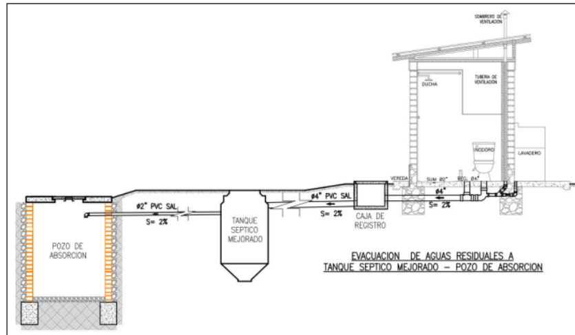
Figura N°08. Vista en corte de los componentes de la UBS con arrastre hidráulico.
