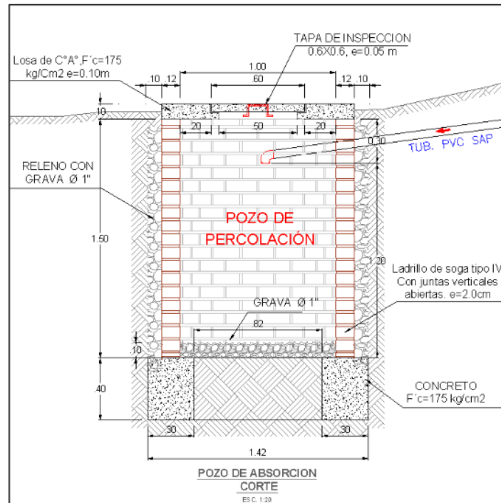
Figura N°14. Plano de pozo de percolación, diseño final. Fuente: Norma técnica de diseño-Opciones Tecnológicas de Saneamiento para el Ámbito Rural.
