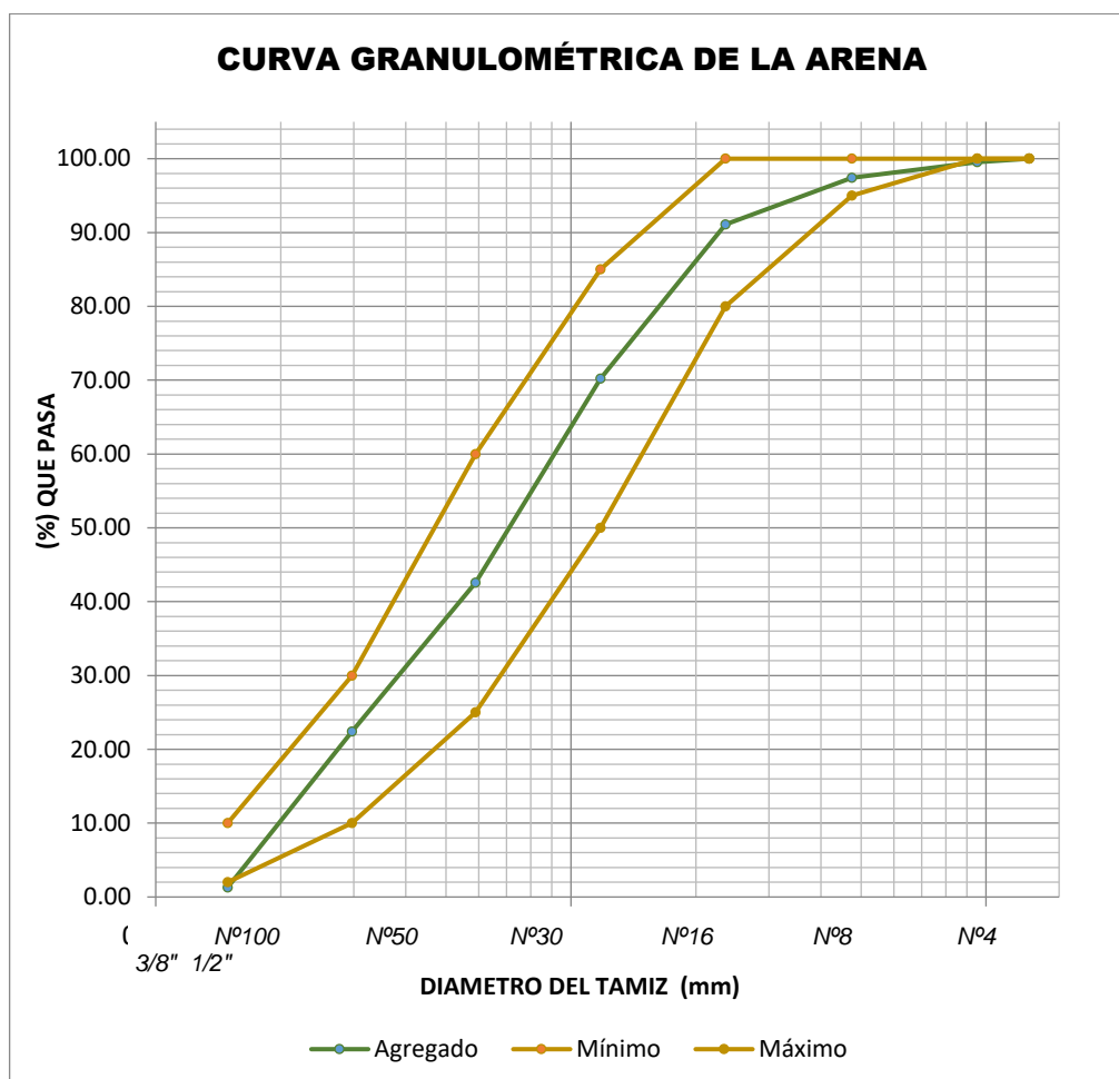
FIGURA 13: CURVA GRANULOMÉTRICA DE LA ARENA
