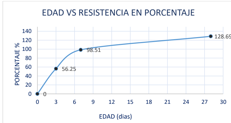
FIGURA 19: EDAD VS RESISTENCIA EN PORCENTAJE MES DE ENERO
