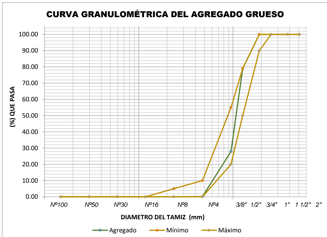
FIGURA 14: CURVA GRANULOMÉTRICA DEL AGREGADO GRUESO
