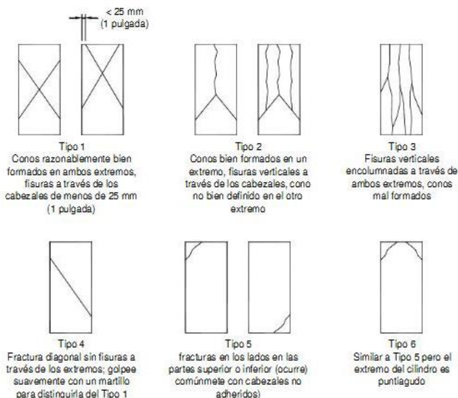
FIGURA 2: TIPOS DE ROTURA DE PROBETAS
