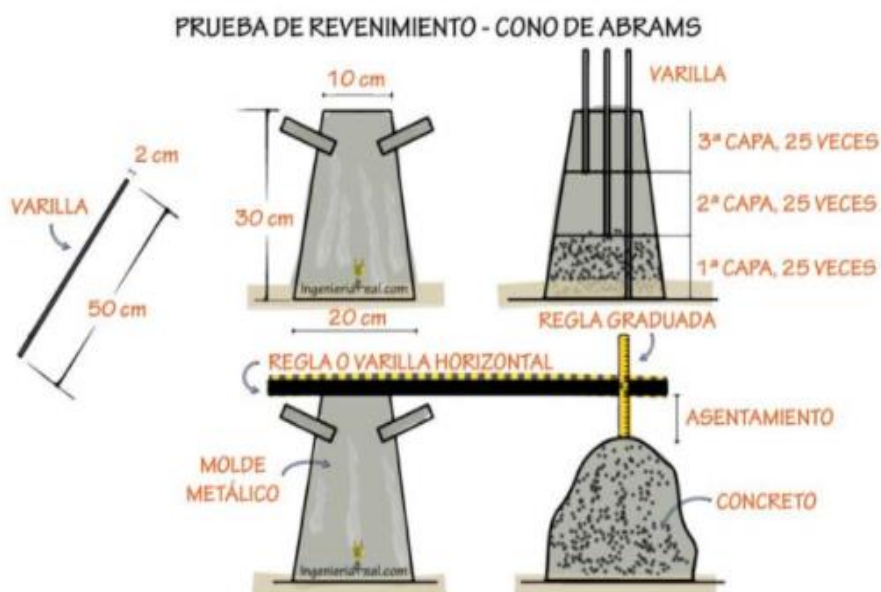
FIGURA 6: PRUEBA DE REVENIMIENTO
