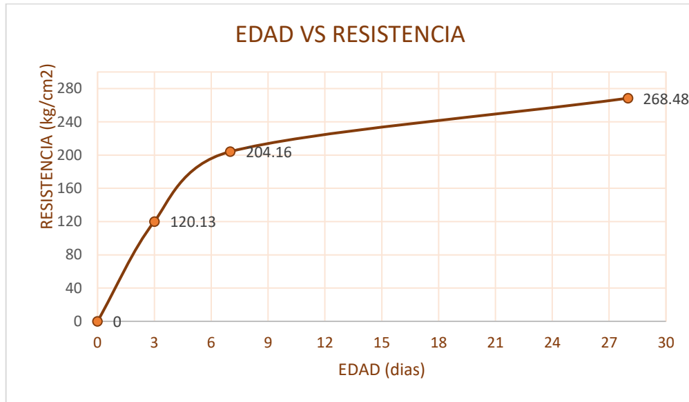
FIGURA 22: EDAD VS RESISTENCIA EN KG/CM 2 MES DE FEBRERO
