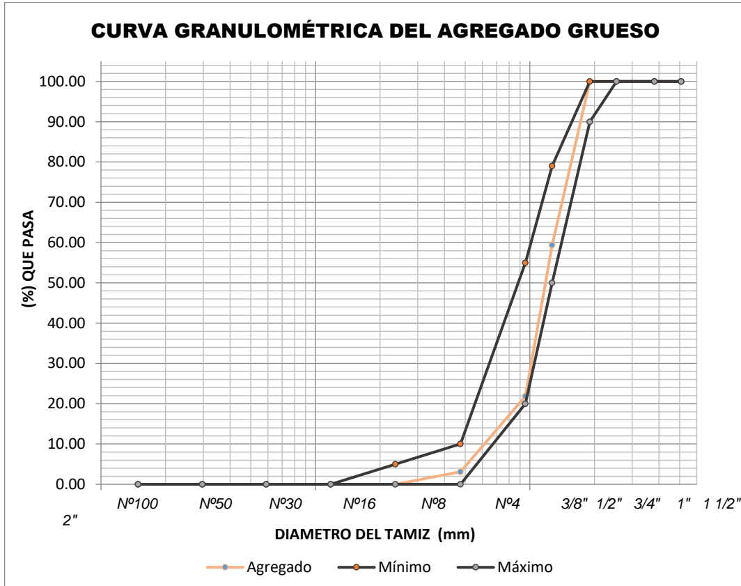
FIGURA 16: CURVA GRANULOMÉTRICA DEL AGREGADO GRUESO
