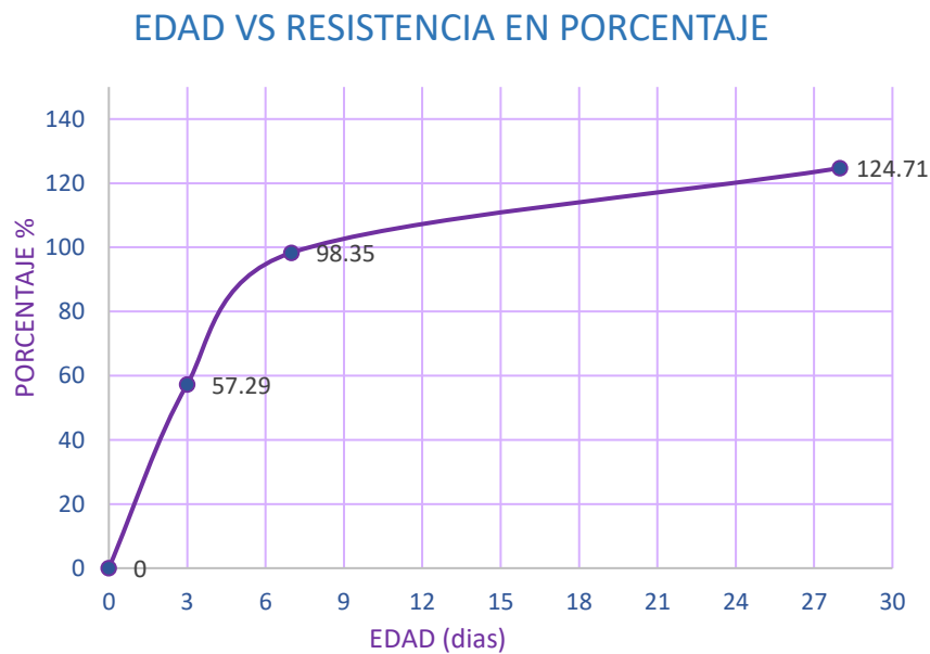
FIGURA 17: EDAD VS RESISTENCIA EN PORCENTAJE MES DE DICIEMBRE
