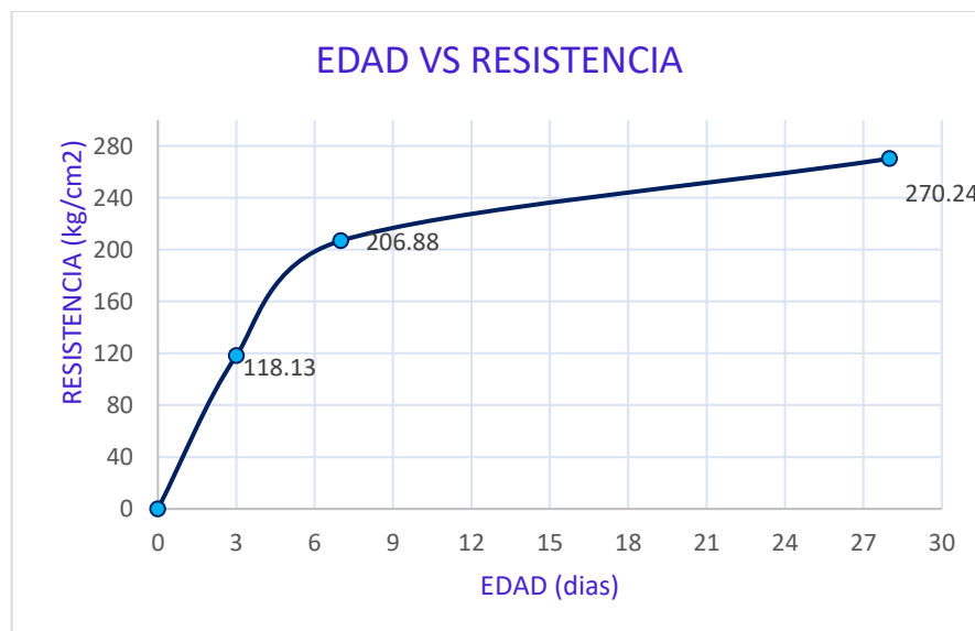
FIGURA 20: EDAD VS RESISTENCIA EN KG/CM 2 MES DE ENERO
