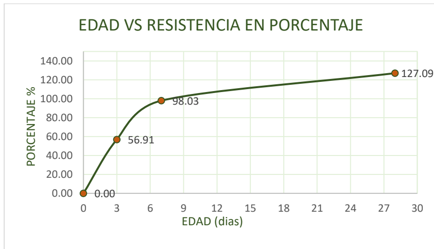
FIGURA 23: EDAD VS RESISTENCIA EN PORCENTAJE GENERAL
