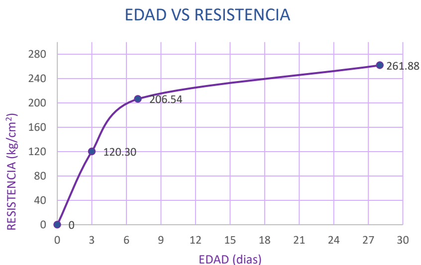
FIGURA 18: EDAD VS RESISTENCIA EN KG/CM 2 MES DE DICIEMBRE
