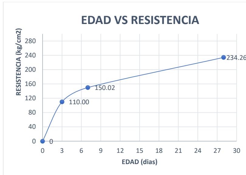
FIGURA 9: RESULTADOS EN RESISTENCIA F'C PROMEDIO
