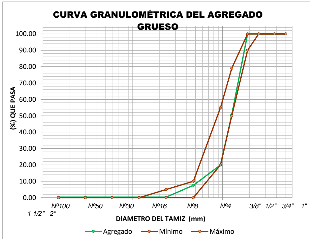
FIGURA 12: CURVA GRANULOMÉTRICA DEL AGREGADO GRUESO
