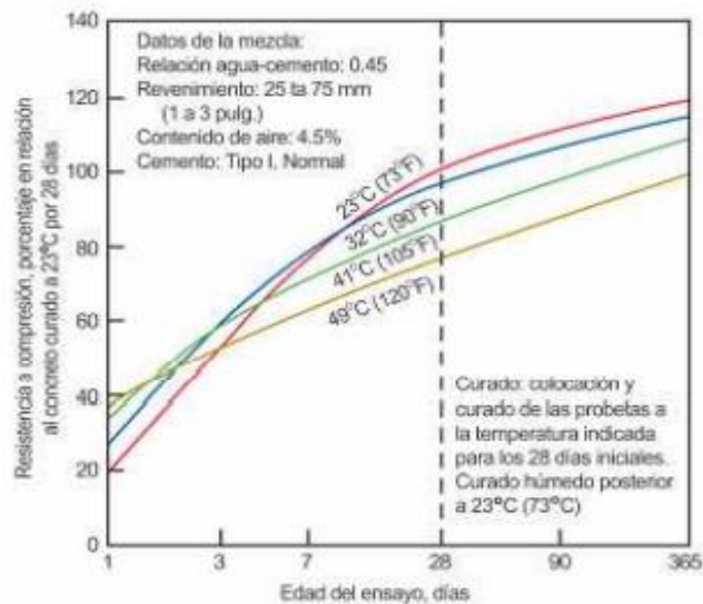
FIGURA 5: SOBRE LA RESISTENCIA
