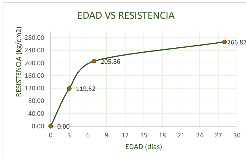
FIGURA 24: EDAD VS RESISTENCIA EN KG/CM 2 GENERAL
