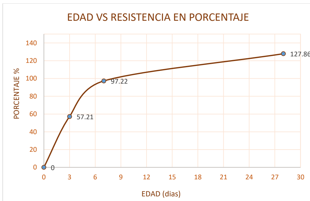
FIGURA 21: EDAD VS RESISTENCIA EN PORCENTAJE MES DE FEBRERO
