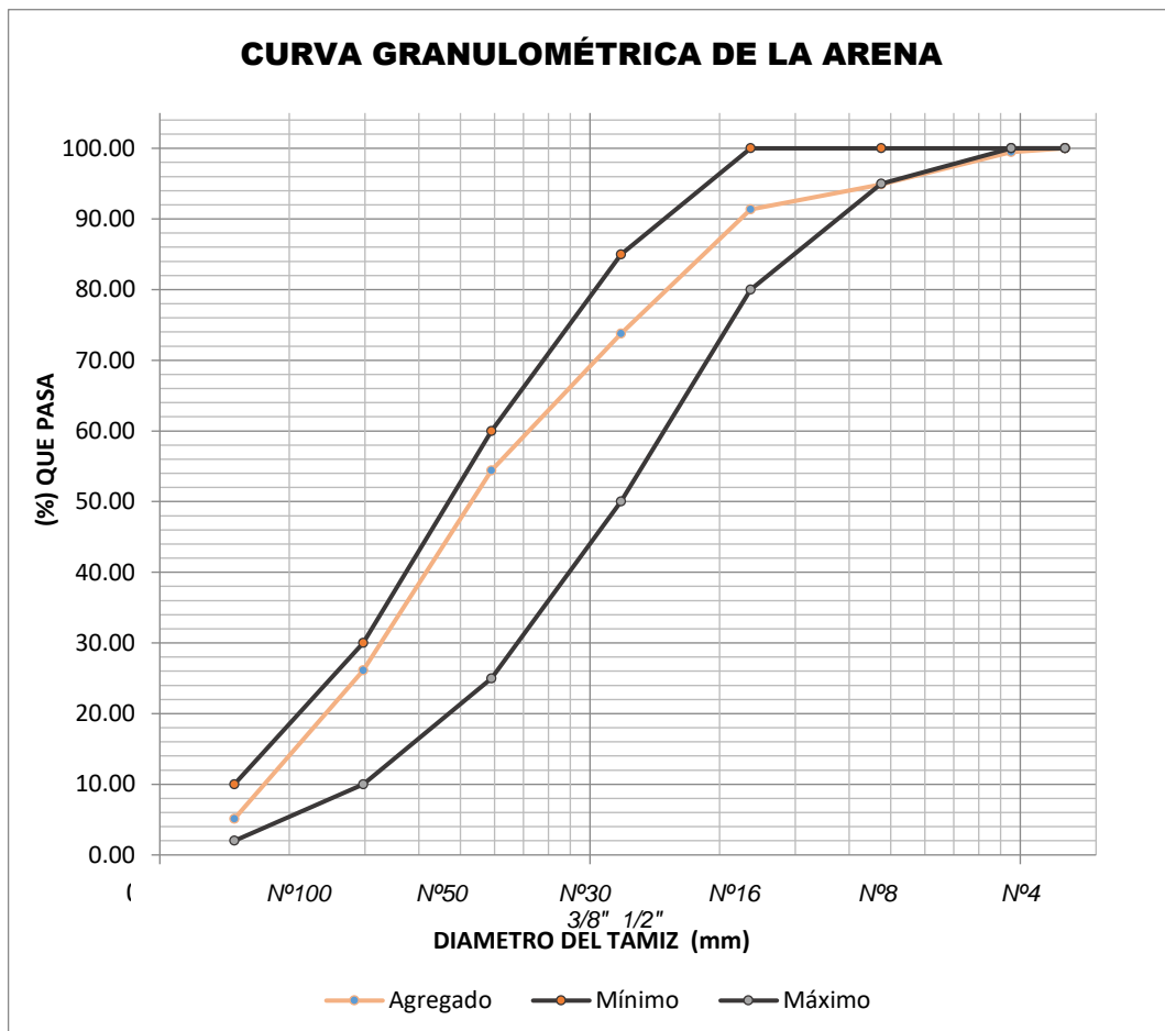
FIGURA 15: CURVA GRANULOMÉTRICA DE LA ARENA
