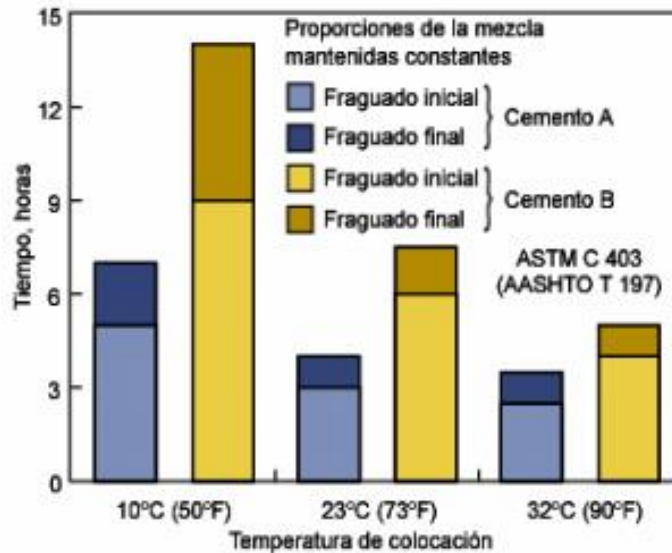
FIGURA 4: SOBRE EL TIEMPO DE FRAGUADO
