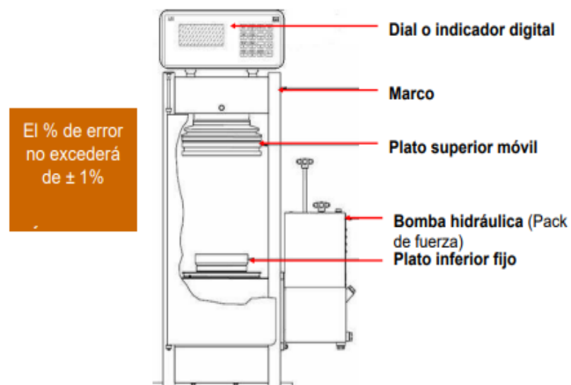
FIGURA 7: PRENSA PARA EL ENSAYO DE RESISTENCIA A LA COMPRESIÓN
