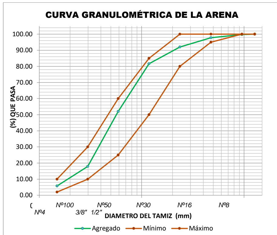
FIGURA 11: CURVA GRANULOMÉTRICA DE LA ARENA
