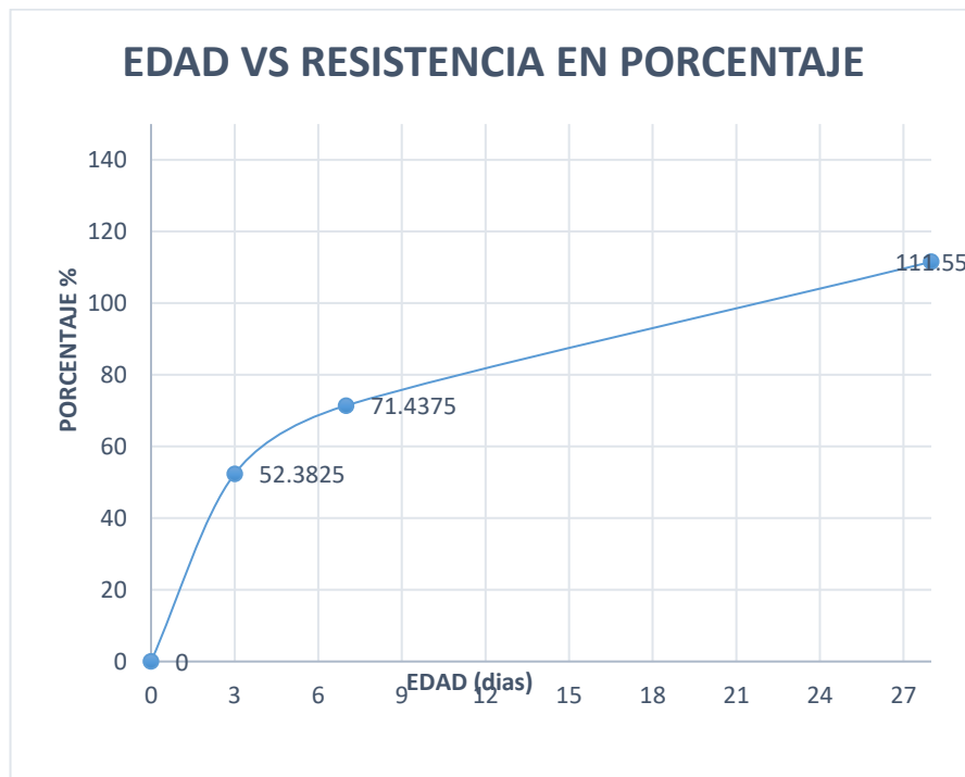
FIGURA 10: RESULTADOS EN PORCENTAJE % PROMEDIO
