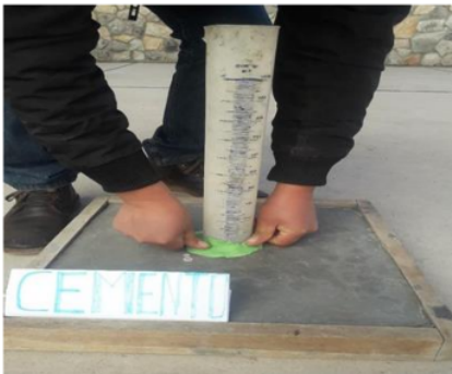
Ensayo de permeabilidad después de la aplicación del impermeabilizante
