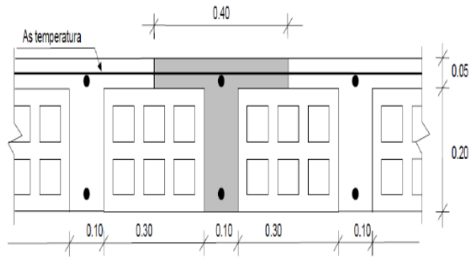
Figura 1 Sección transversal de una losa aligerada Fuente: Elaboración propia.
